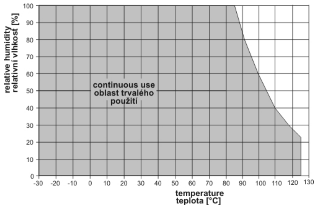
Obrázek: Provozní rozsah snímače vlhkosti
