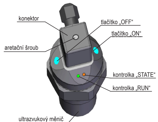
Popis hlavních částí snímače verze s tlačítky
