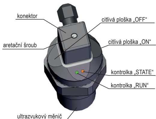
Popis hlavních částí snímače verze s hallovými sondami
