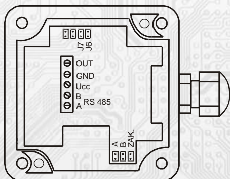
Rozmístění připojovacích svorek a jumperů (obr.1):
