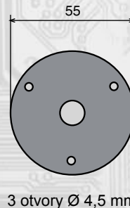
Držák středový A - pro P12F
