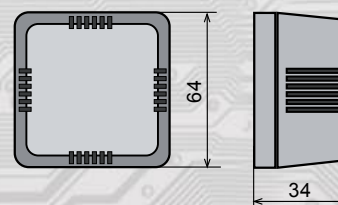
Snímač do interiéru - P10F
