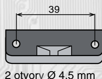
Držák boční A - pro P11F
