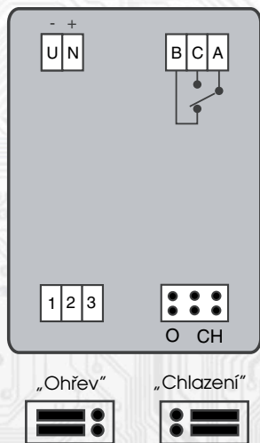
Zapojení Pt100
