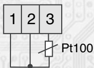
Zapojení Pt100
